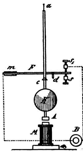
Č. 1738. Hippovy vlastní elektrické hodiny.
